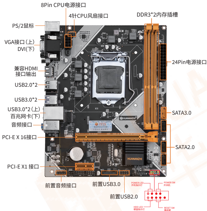
图1-1 B75主板图解
