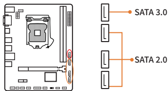
图2-9 SATA接口
