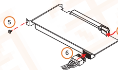
图2-8 显卡安装
