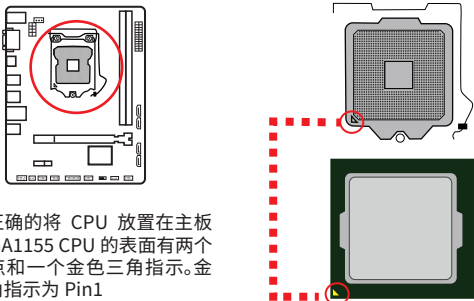
图2-6 CPU安装
