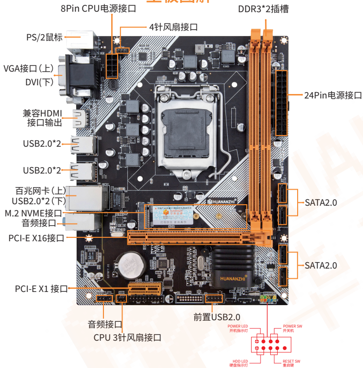
图1-1 H61主板图解
