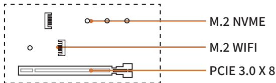
图2-4 PCI扩展插槽
