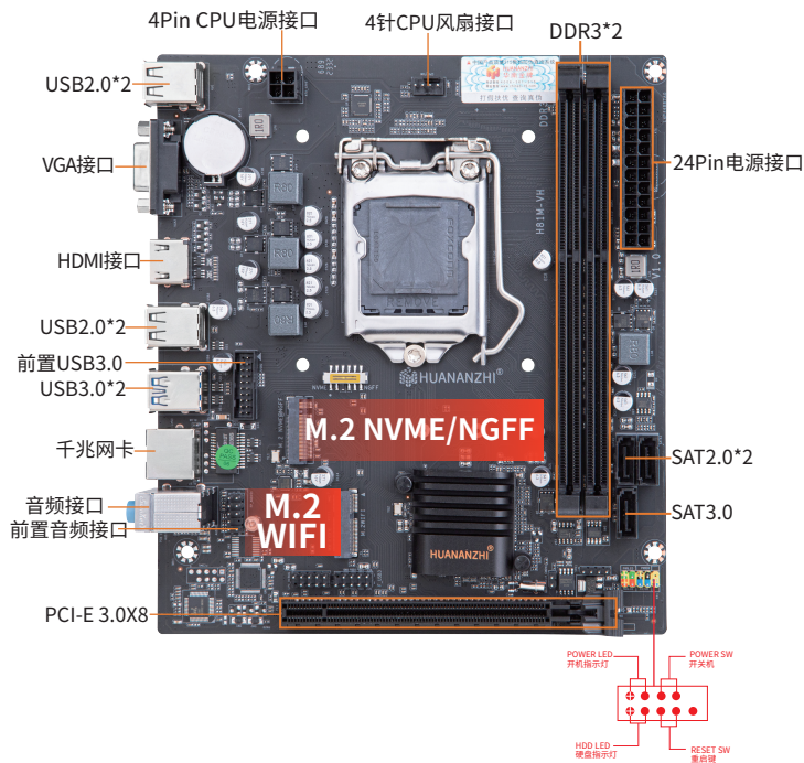
图1-1 H81M-VH主板图解
