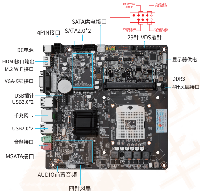
图1-1 HM65M-I 主板图解
