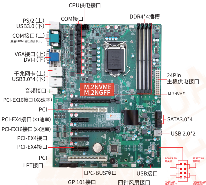
图1-1 Q170主板图解
