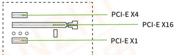
图2-4 PCI扩展插槽
