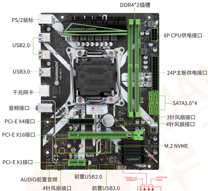
图1-1 X99-8M F主板图解
