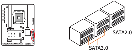
图2-11 SATA接口
