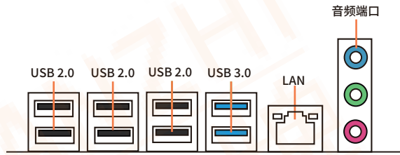
图1-2 整体后置I/O面板展示
