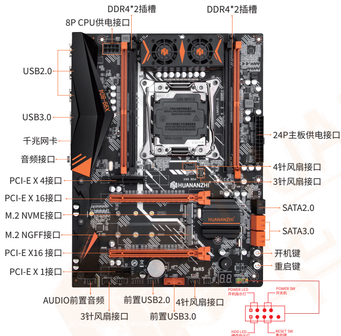
图1-1 X99-BD4主板图解
