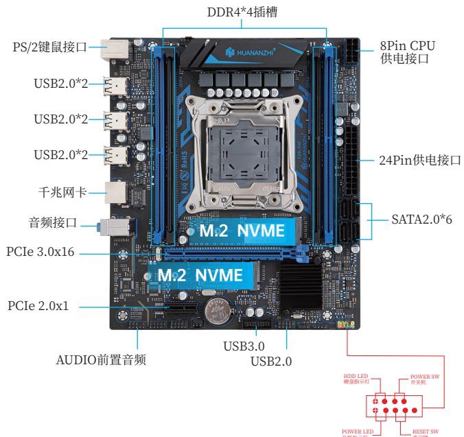
图1-1 X99-P4F主板图解
