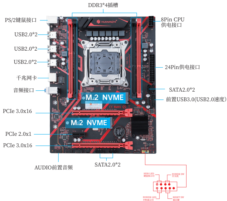
图1-1 X99-PD3主板图解
