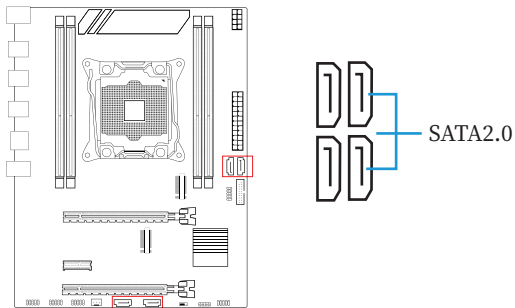
图2 -11 SATA接口
