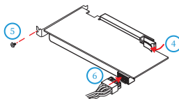
图2-10 显卡安装
