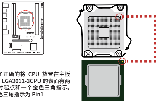
图2-7 CPU安装
