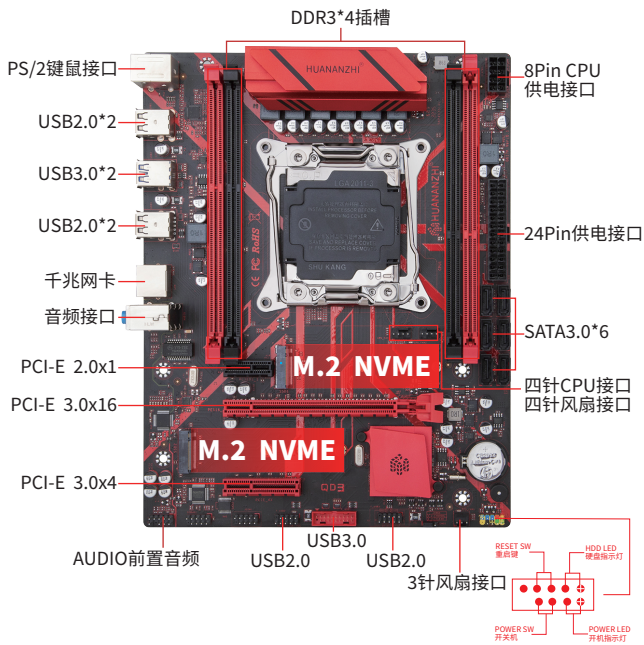
图1-1 X99-QD3主板图解
