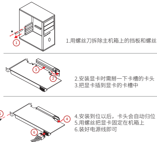
图2-10 显卡安装
