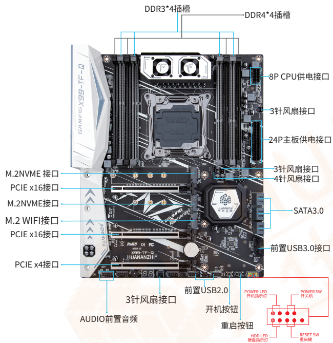
图1-1 X99-TF-Q 主板图解
