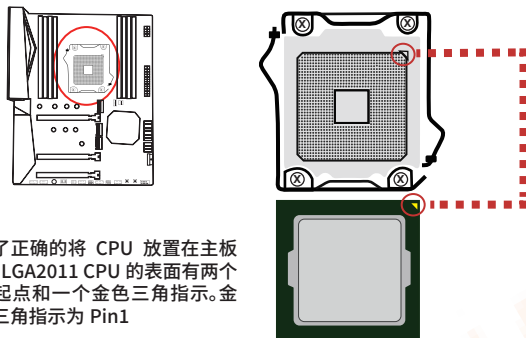
图2-7 CPU安装
