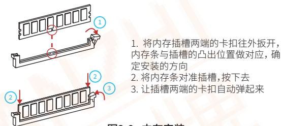
图2-9 内存安装
